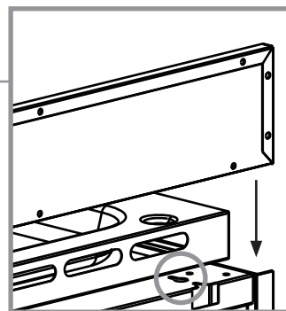
Détail de l'emplacement du « trou de serrure »
